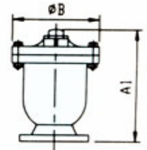
FIG.412 FLANGE END
